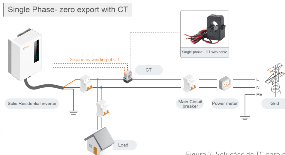
Figura 2: Soluções de TC para sistemas monofásicos
