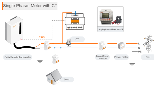
Medidor com TC
