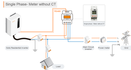
Medidor sem TC
