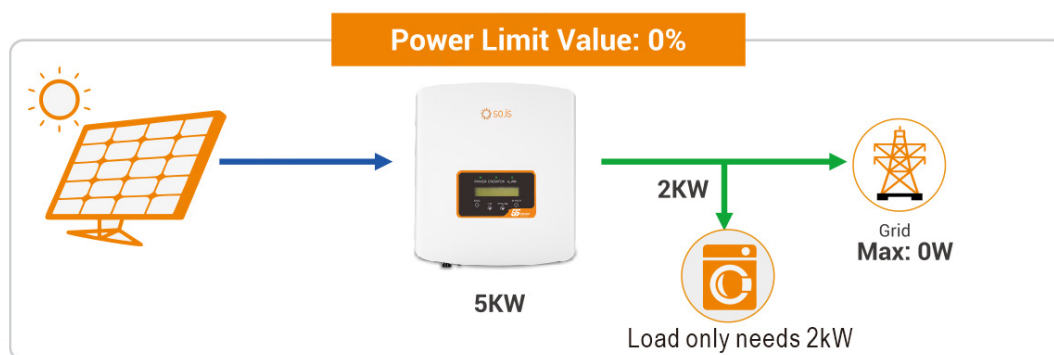
Figura 1: Limitação de injeção zero
