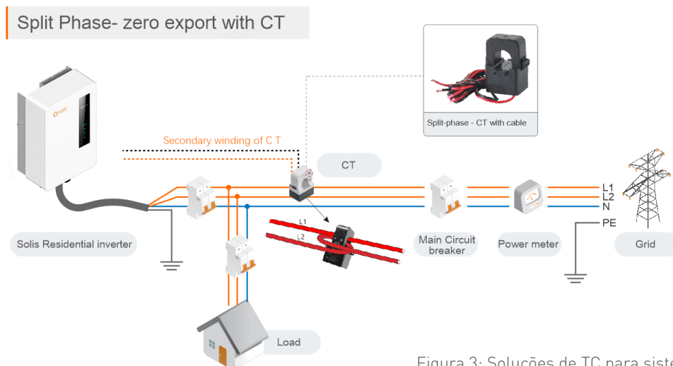
Figura 3: Soluções de TC para sistemas de fase dividida
